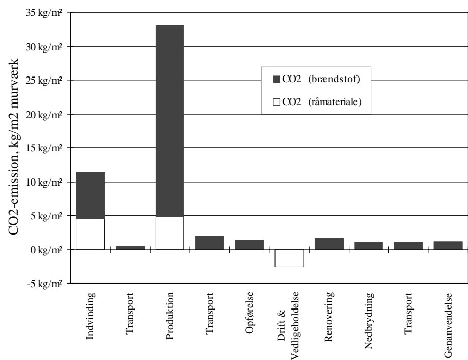
Figur 0.11 Totalt CO 2 -emission for 1 m 2 mureværk indenfor mureværkets 1. leveår. I opgørelsen er anvendt vægtet gennemsnit for indvinding af ler, sand, teglsten og mørtel.
