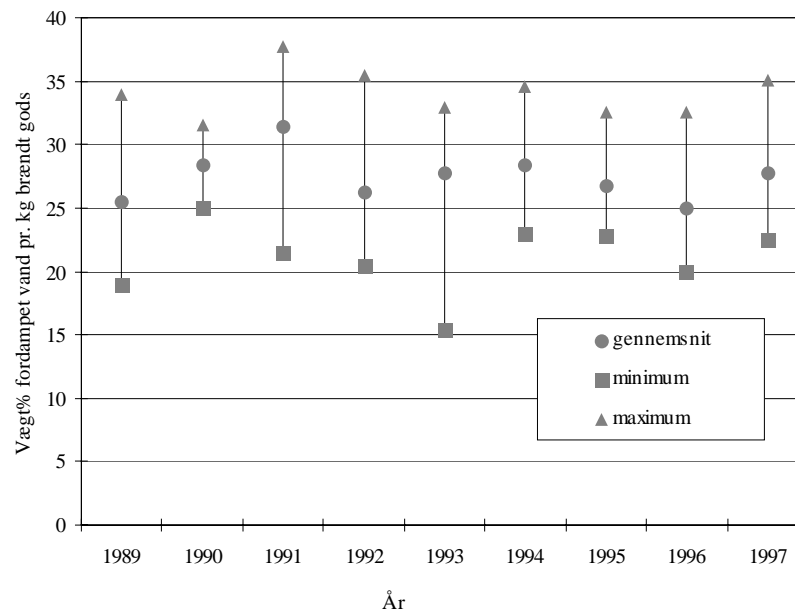
Figur 0.3 Gennemsnitlig mængde vand der borttørres.
